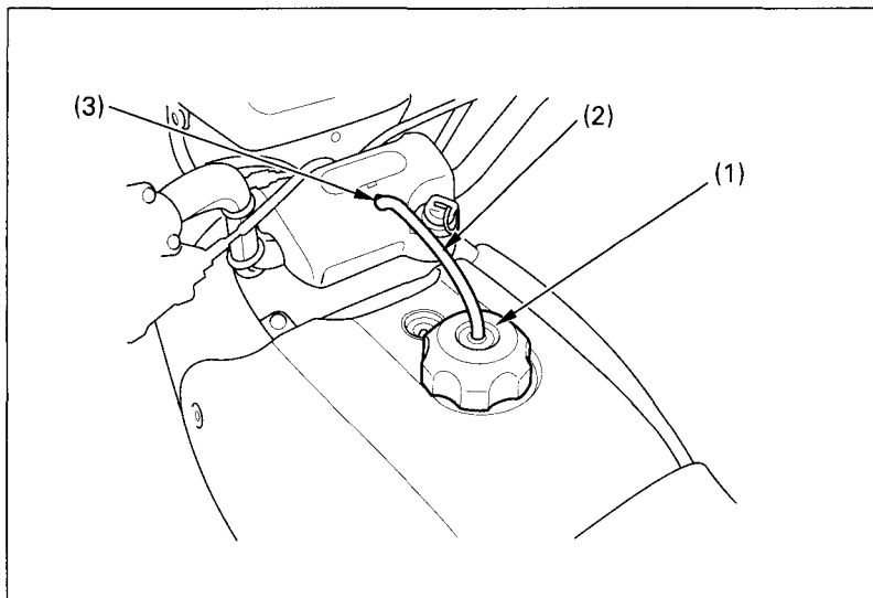
Fig. 2-26 (1) Fuel fill cap
