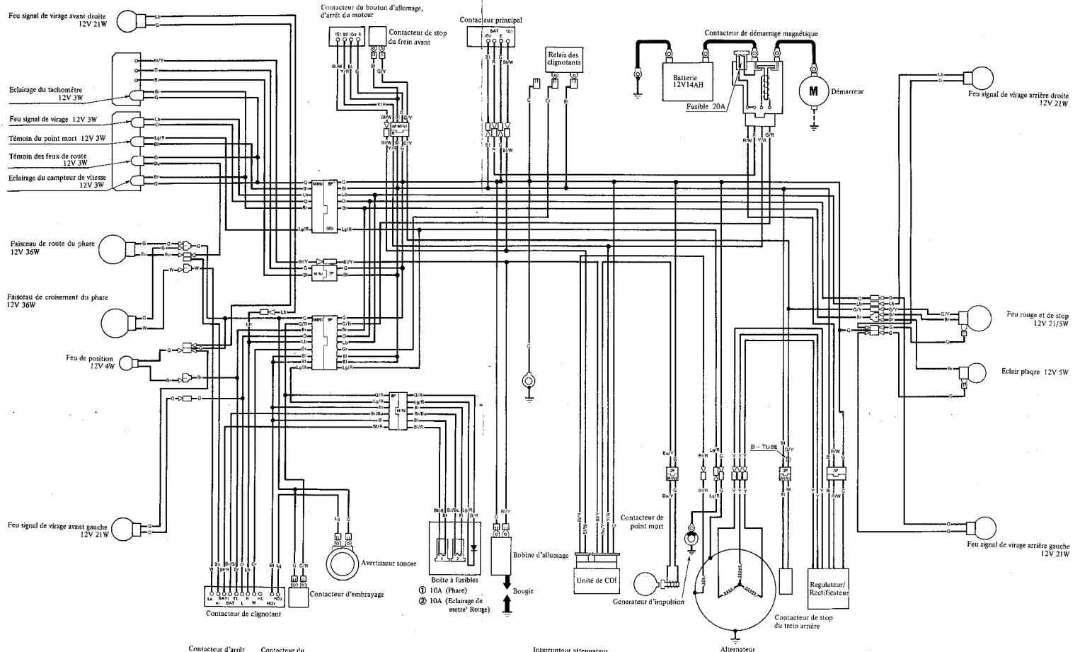
Contacteur d'avertisseur
