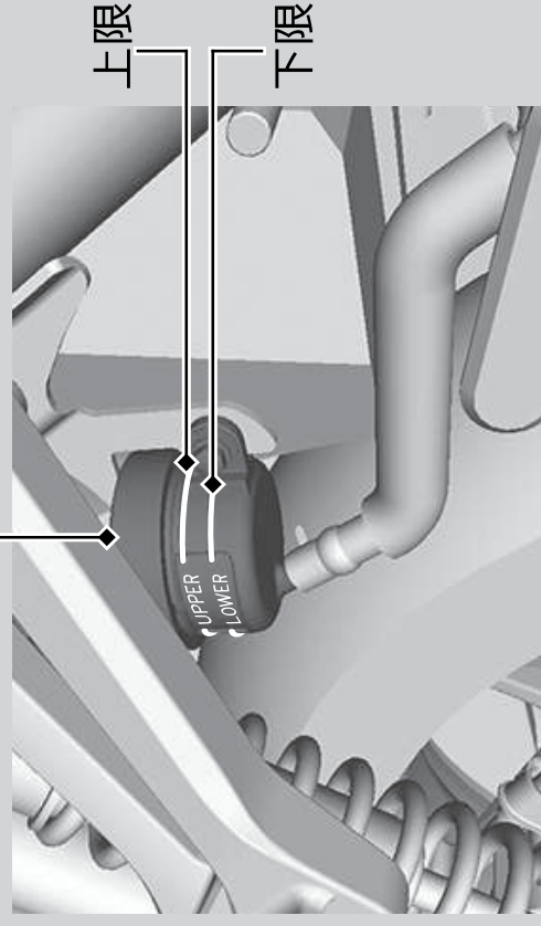
後輪ブレーキリザーバータンク
