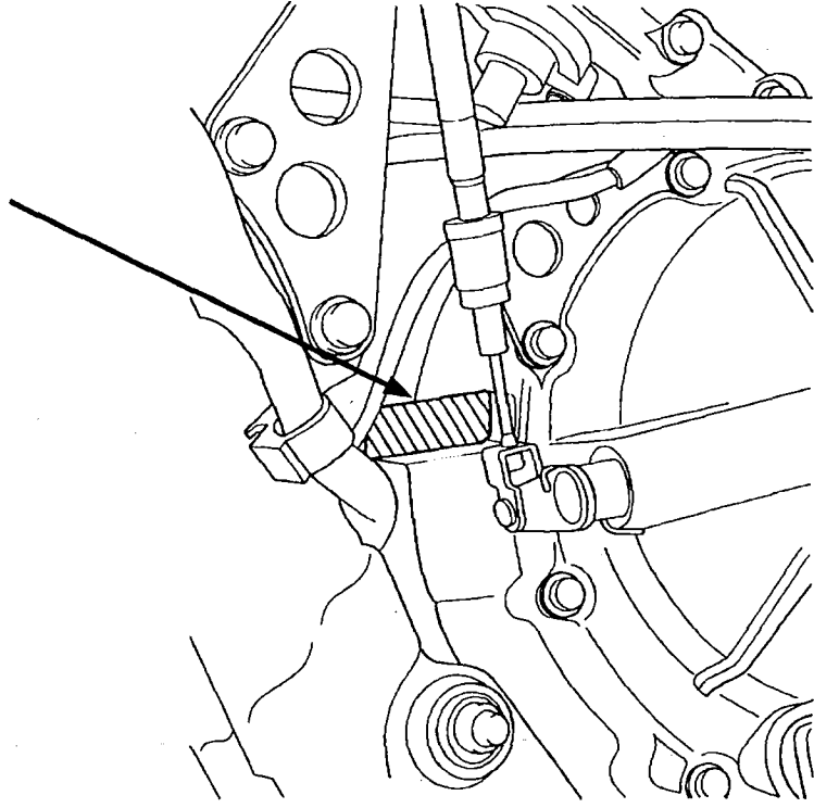
エンジン号機打刻位置
