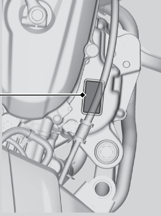
エンジンナンバー打刻位置
